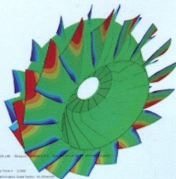
特种叶轮转子叶型的数字化分析
